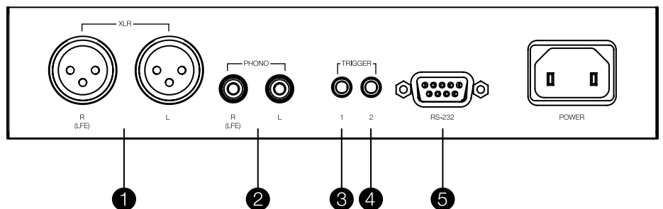
다이어그램 3 DB 서브우퍼 연결 패널
