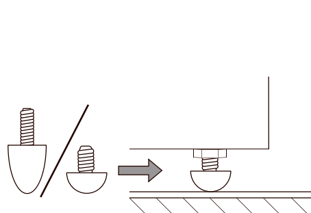
Diagrama 2b Uso de los pies de desacoplo y los pies de goma
